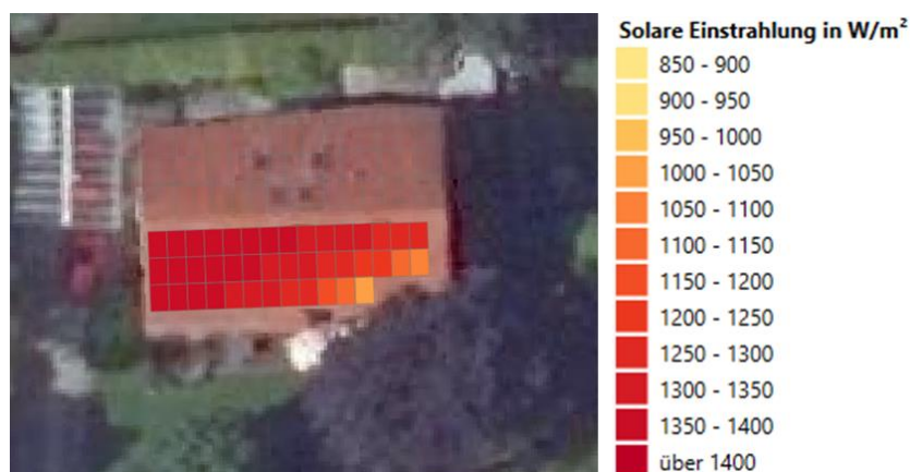
Abbildung 20: Beispielgebäude mit modelliertem Dach-Photovoltaikpotenzial und Einstrahlungswerten pro Modul.
