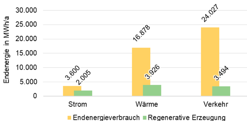
Abbildung 13: Gegenüberstellung von Energieverbrauch und Erzeugung in den Sektoren Strom, Wärme und Verkehr.
