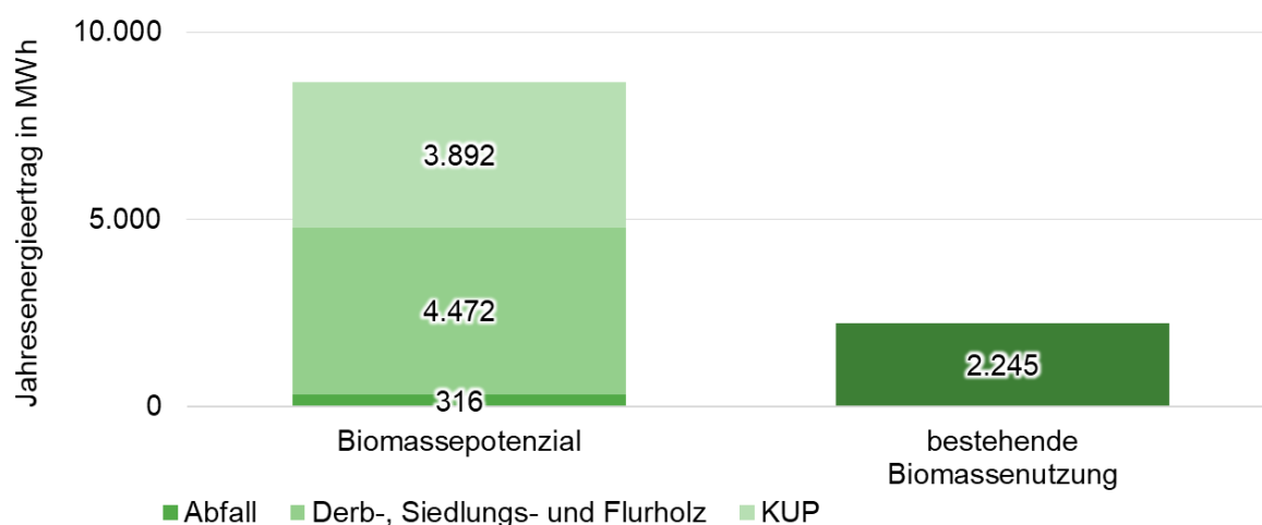
Abbildung 23: Potenzial zur Energieerzeugung aus Biomasse.
