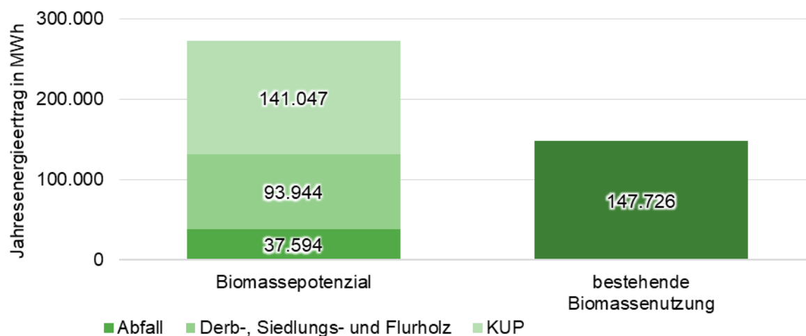
Abbildung 25: Summiertes Potenzial zur Energieerzeugung aus Biomasse im Landkreis Fürstentfeldbruck.
