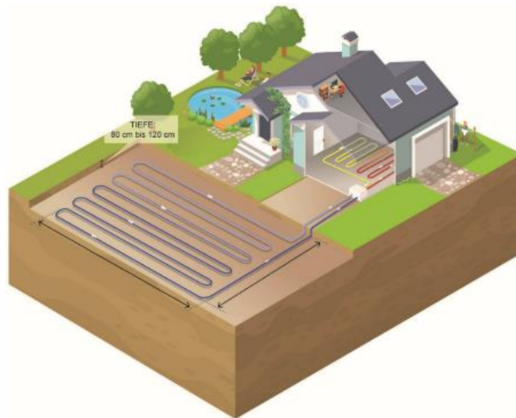
Abbildung 29: Der typische Aufbau eines Erdwärmekollektors (Bildquelle: Interreg Alpine Space Programme, Projekt GRETA).
