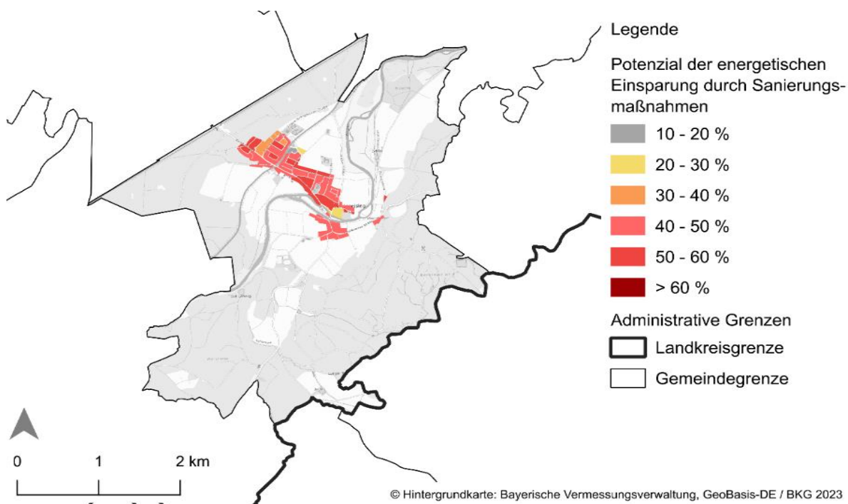
Abbildung 17: Einsparungspotenzial im Wärmesektor für Wohngebäude mit Sanierungsszenario "Mittel".
