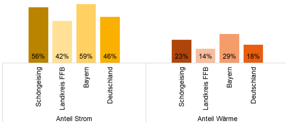
Abbildung 15: Anteil der erneuerbaren Energien am Bruttostromverbrauch und an der Wärmebereitstellung im Jahr 2022 im überregionalen Vergleich (Datenquelle für überregionale Werte: StMWi, BMWK).
