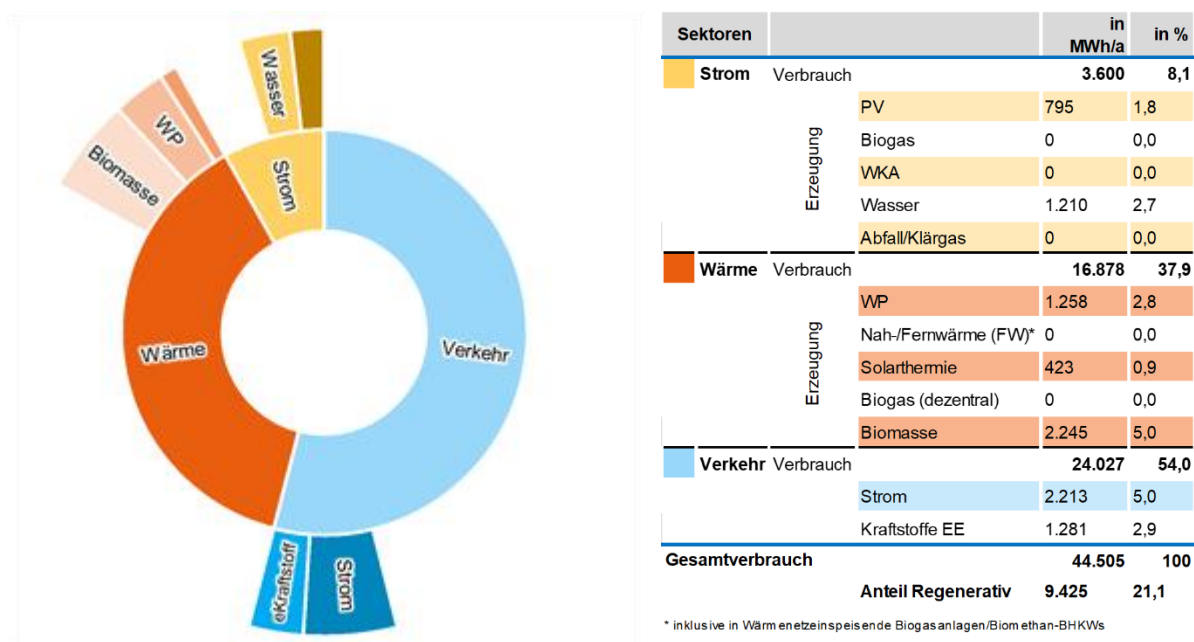
Abbildung 14: Vergleich der erneuerbaren Energieerzeugung und des Verbrauchs im Jahr 2022. 15
