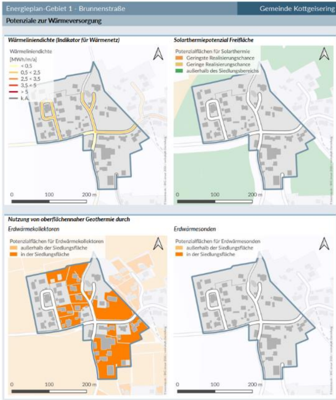
Abbildung 5-4: Kartografische Darstellungen Wärmelinienichte, der Solarthermiepotenziale auf Freiflächen sowie der Potenziale für Erdwärmesonden und Erdwärmekollektoren
