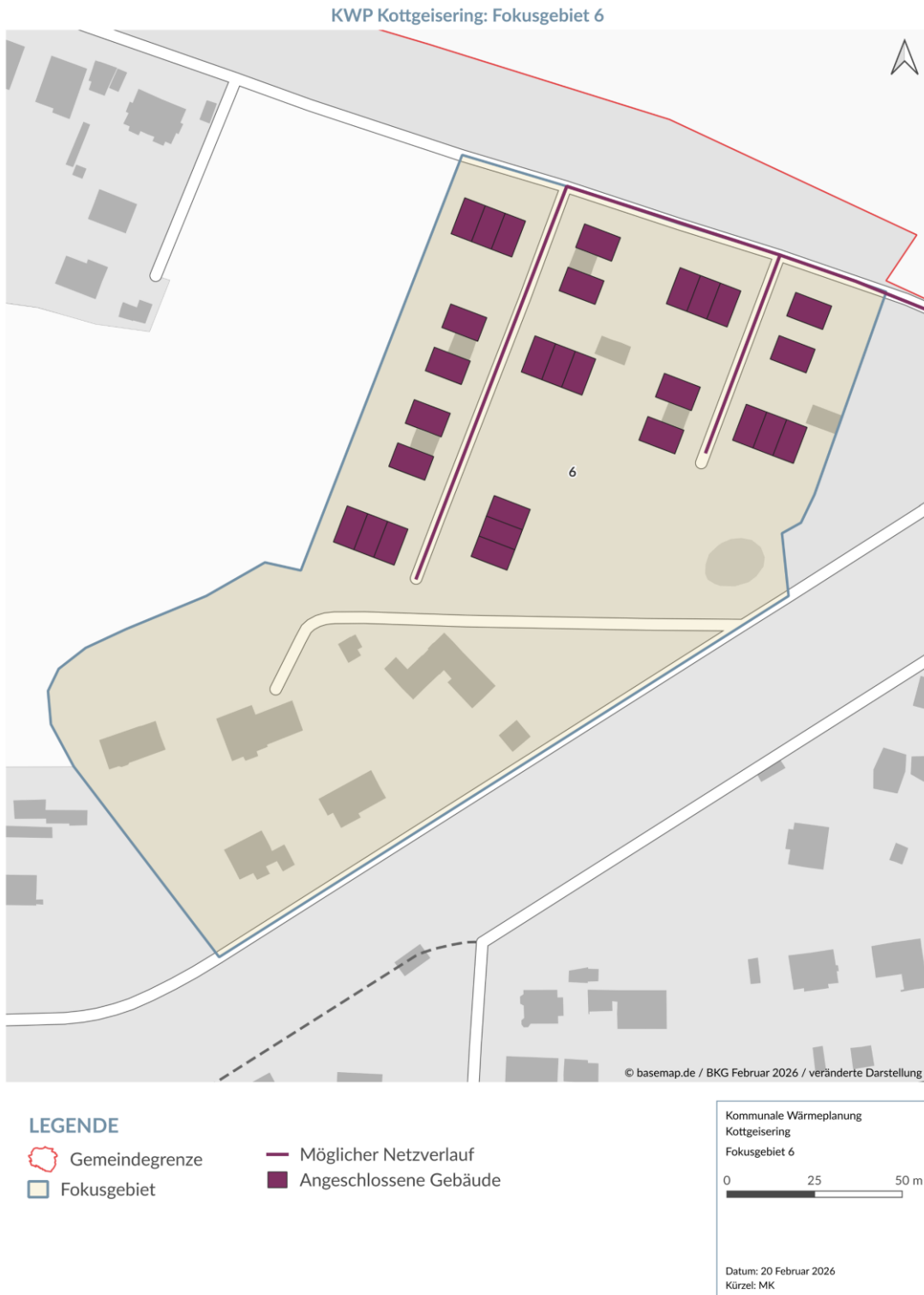
Abbildung 5-9: Möglicher Trassenverlauf des Wärmenetzes im Teilgebiet 6
