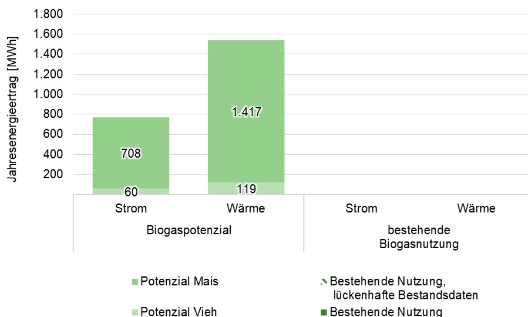
Abbildung 25: Potenzial zur Energieerzeugung durch Biogasanlagen. 32
