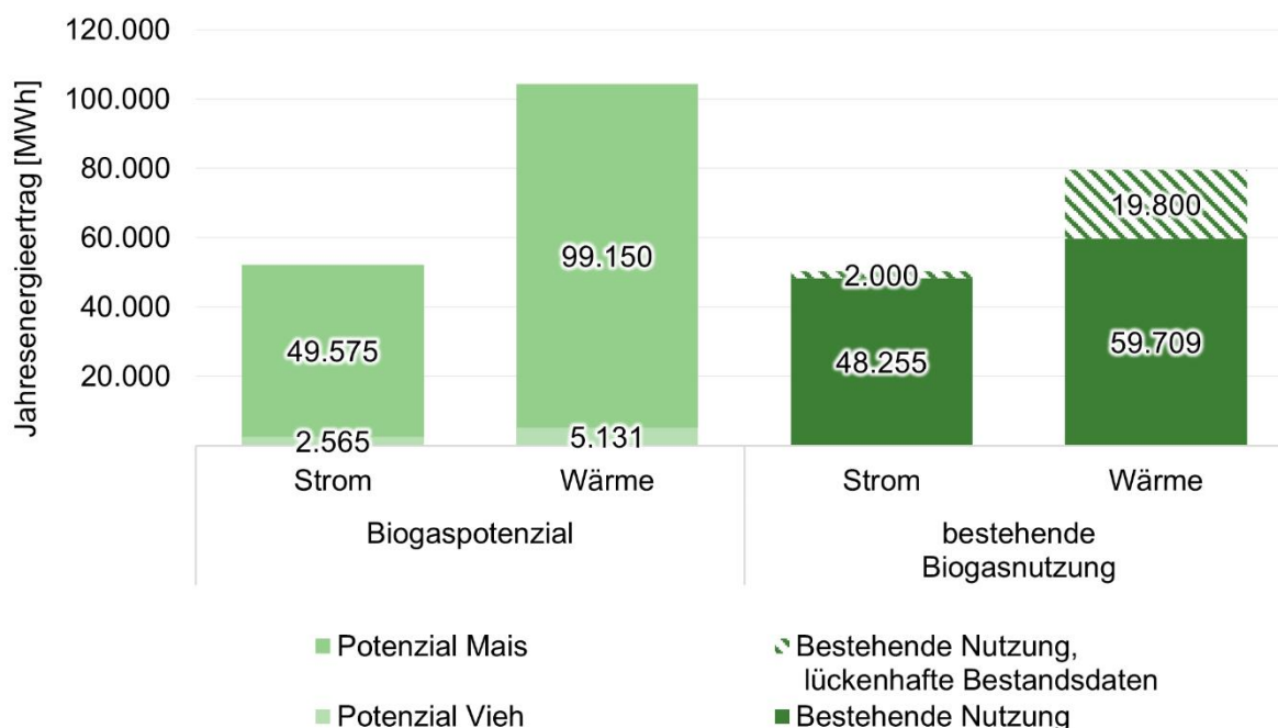
Abbildung 27: Summiertes Potenzial zur Energieerzeugung aus Biogas im Landkreis Fürstfeldbruck.
