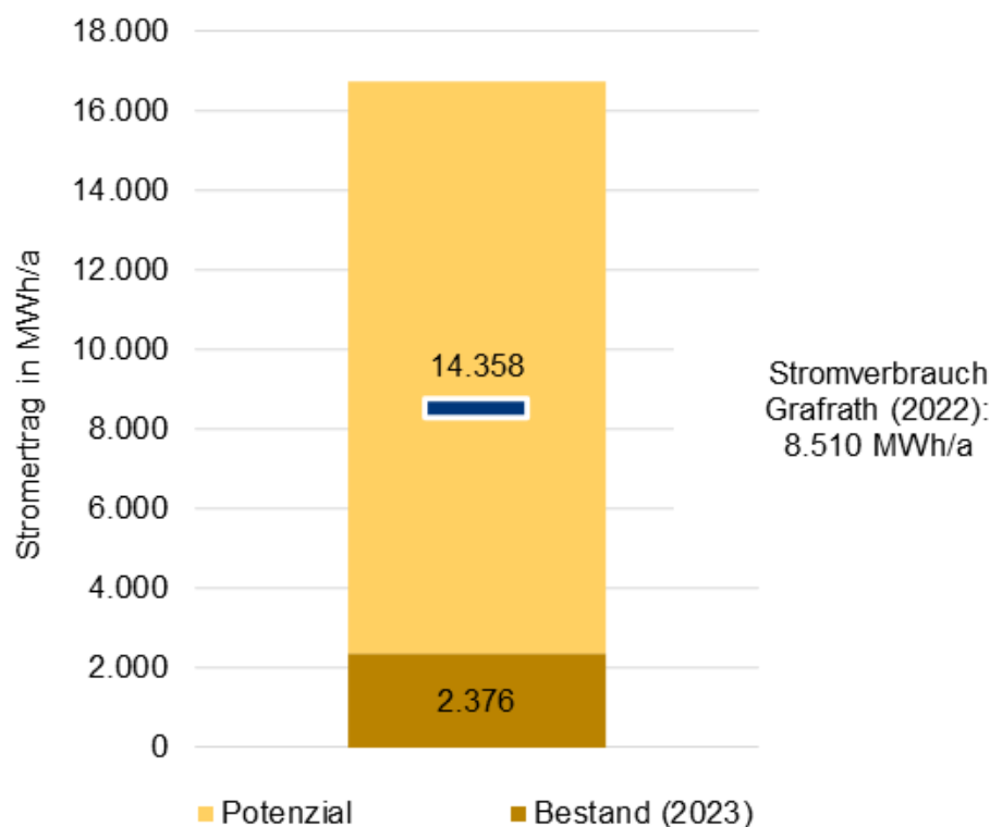
Abbildung 22: Ausbaupotenzial für Dach-Photovoltaikanlagen.
