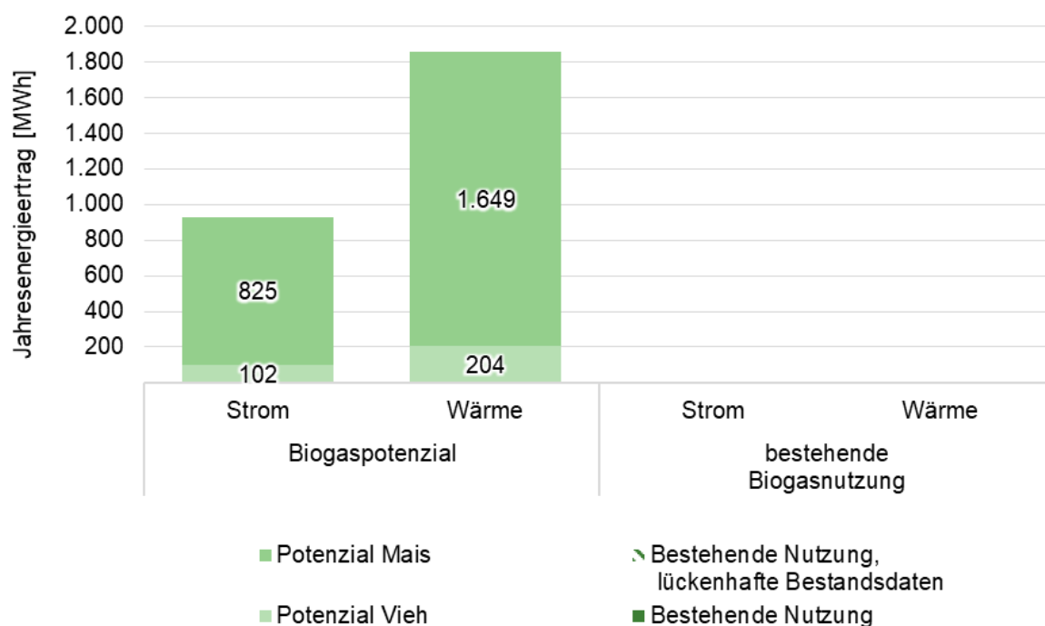
Abbildung 25: Potenzial zur Energieerzeugung durch Biogasanlagen. 32
